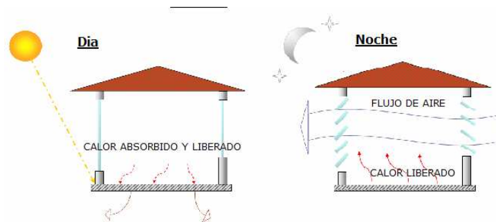
Figura 3 : Esquema del funcionamiento de la Masa Térmica del Hormigón en VERANO
