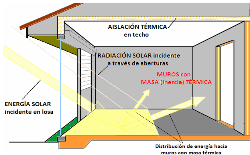
FIGURA 2: Incidencia de la energía solar en distintos elementos que integran la envolvente de una vivienda.
