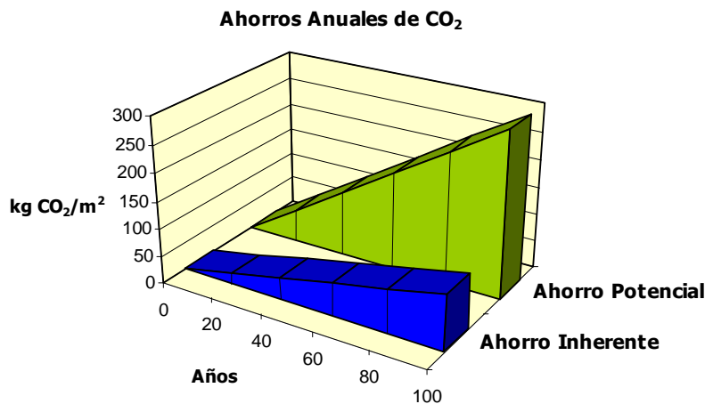
FIGURA 6: Ahorros de CO 2 por Masa Térmica (3)
