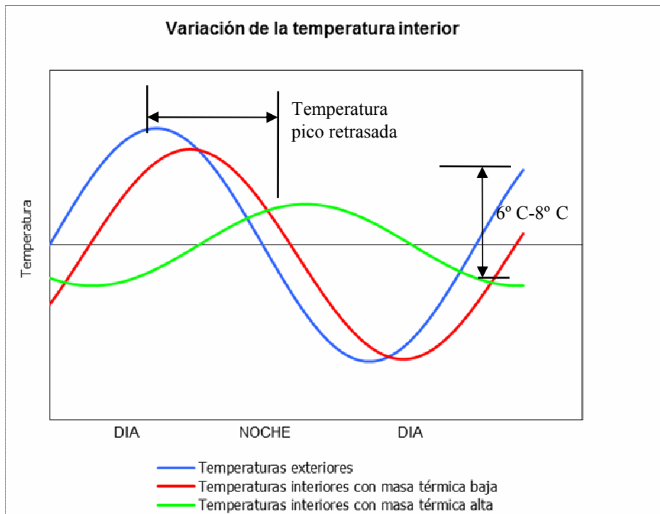
FIGURA 5: Evolución diaria de las temperaturas
